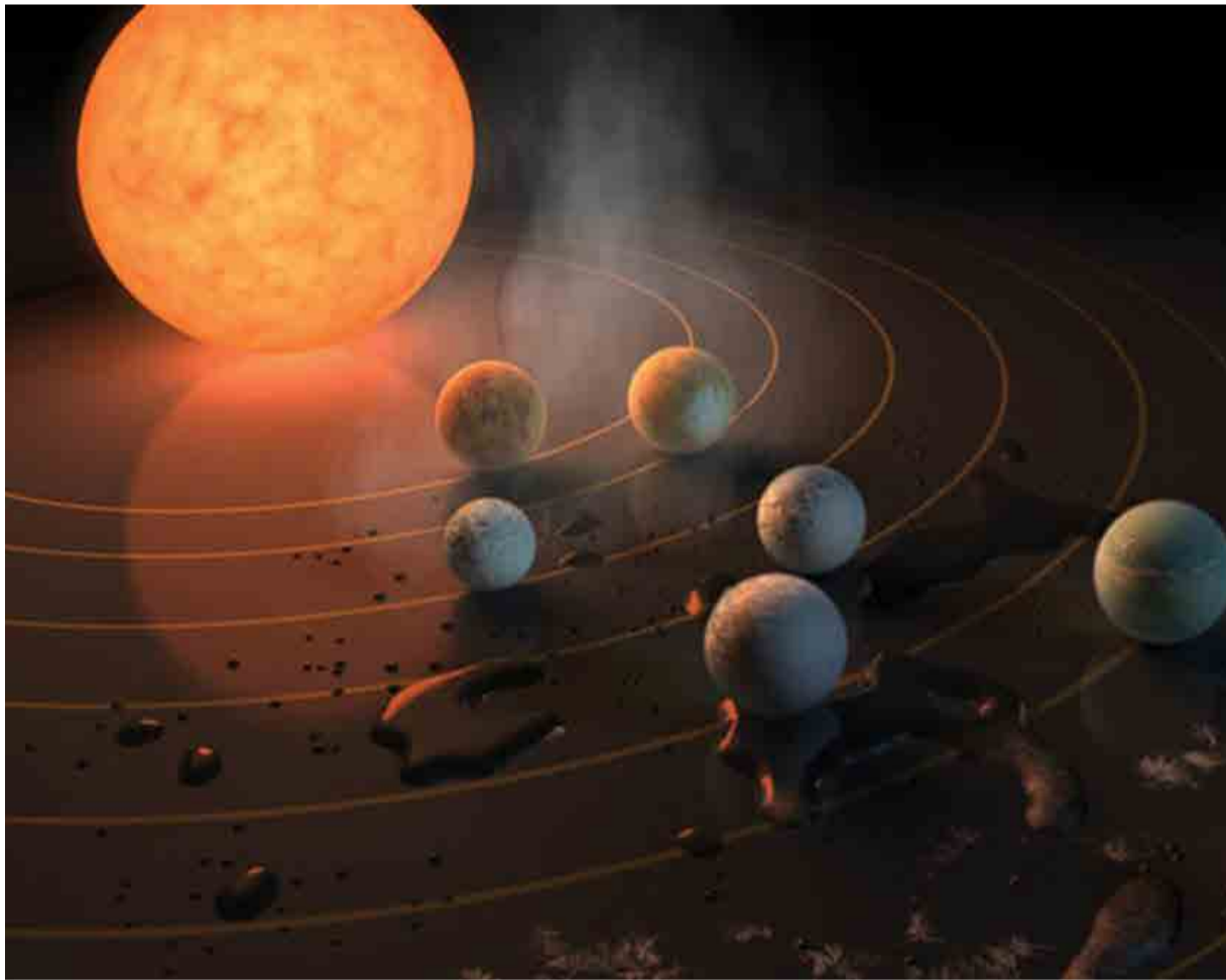
Trappist-1 гарагийн атмосфер дэх хүчилтөрөгч, метан, нүүрсний давхар исэл болон усны илрэл нь биологийн идэвхжиллийн нотолгоо байж болох юм.
